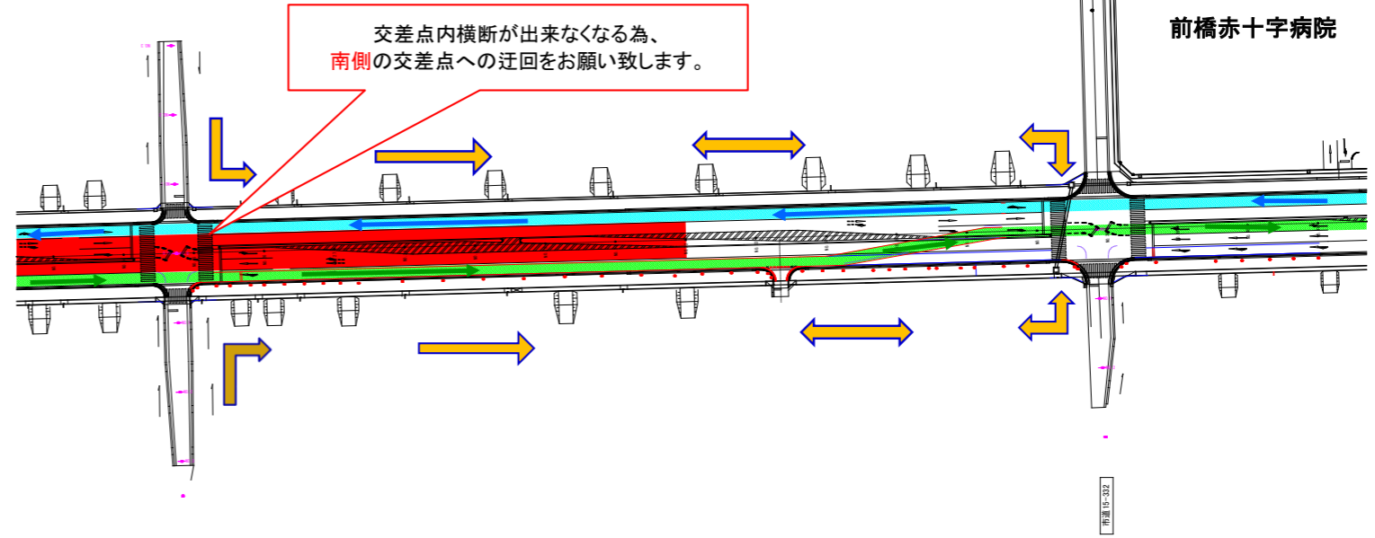
【迂回路計画図】
